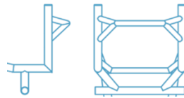
Stabilisation bar, type X
